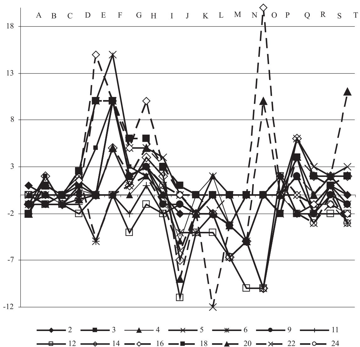
Рис. 1. Нормированные отклонения признаков цветков Salvia officinalis L. (А – Т, см. табл.) относительно контроля в значении «0»: 2 – 24 – образцы
