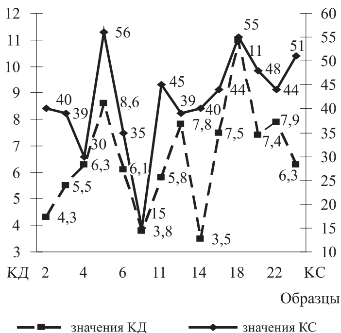
Рис. 3 Коэффициенты дивергенции (КД) и семинификации (КС) образцов Salvia officinalis L. (№ 1 – 24)
