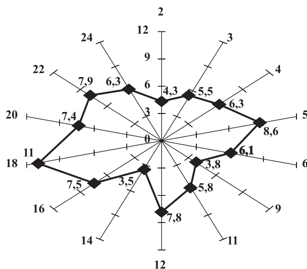
Рис. 2. Коэффициенты дивергенции по комплексу признаков Salvia officinalis L. относительно контроля в значении «0»: 2 – 24 – образцы
